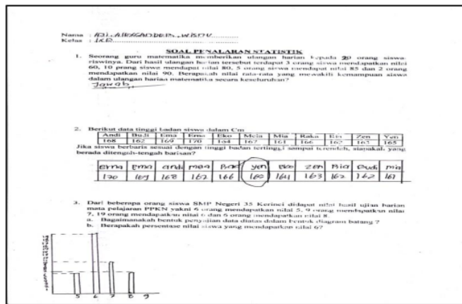
Gambar 1. Siswa menjawab soal penalaran statistis yang diberikan.
